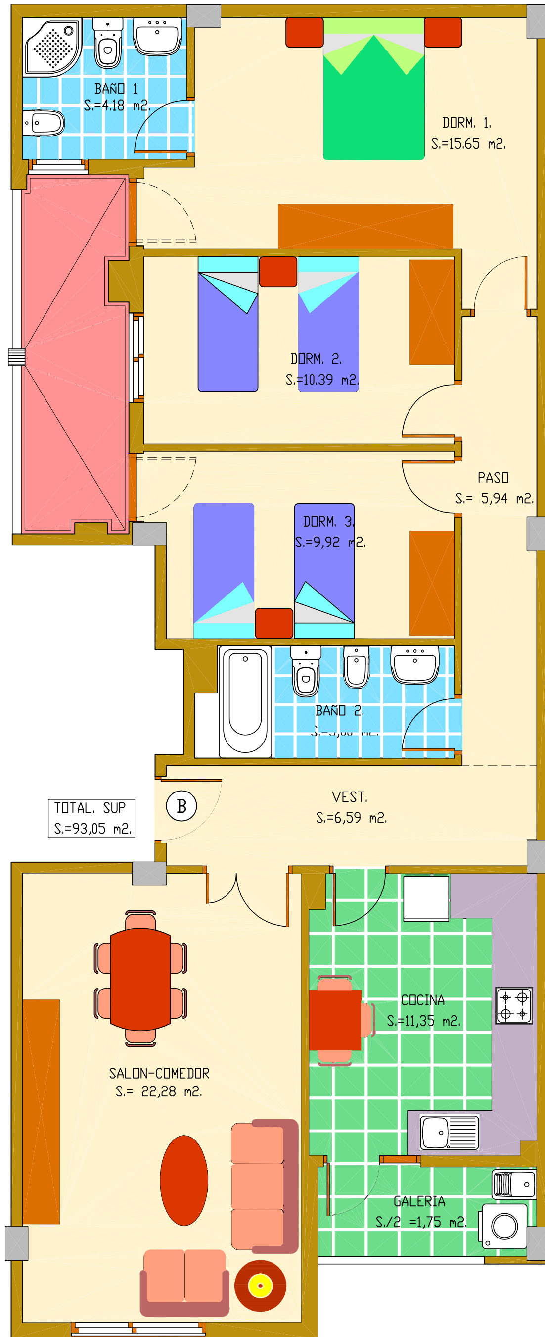
VIVIENDA TIPO B PLANTA DE PISO 1º
